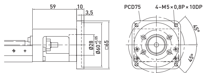
Adapter flange F10
